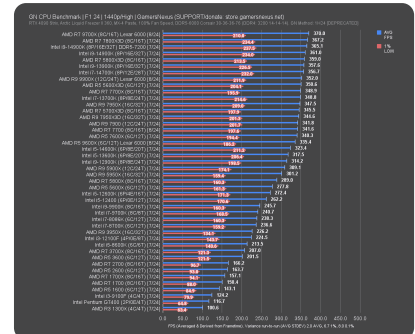
F1 2024 1080p & 1440p CPU Benchmarks.
